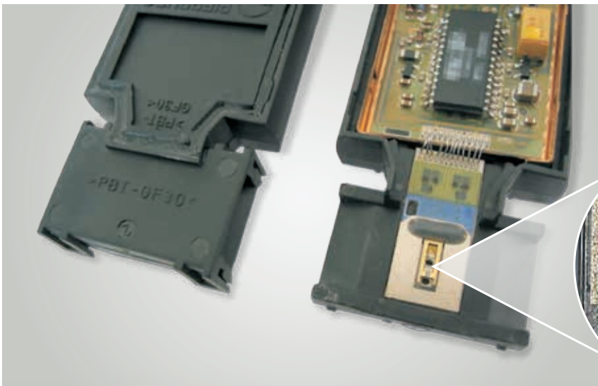
Ölnebel auf Heißfilmsensor
